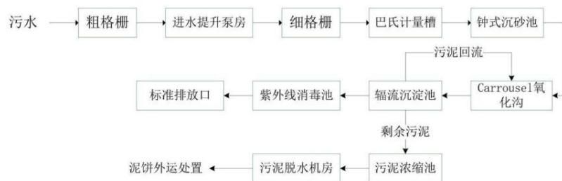
图 4-1 污水处理厂处理工艺流程图
