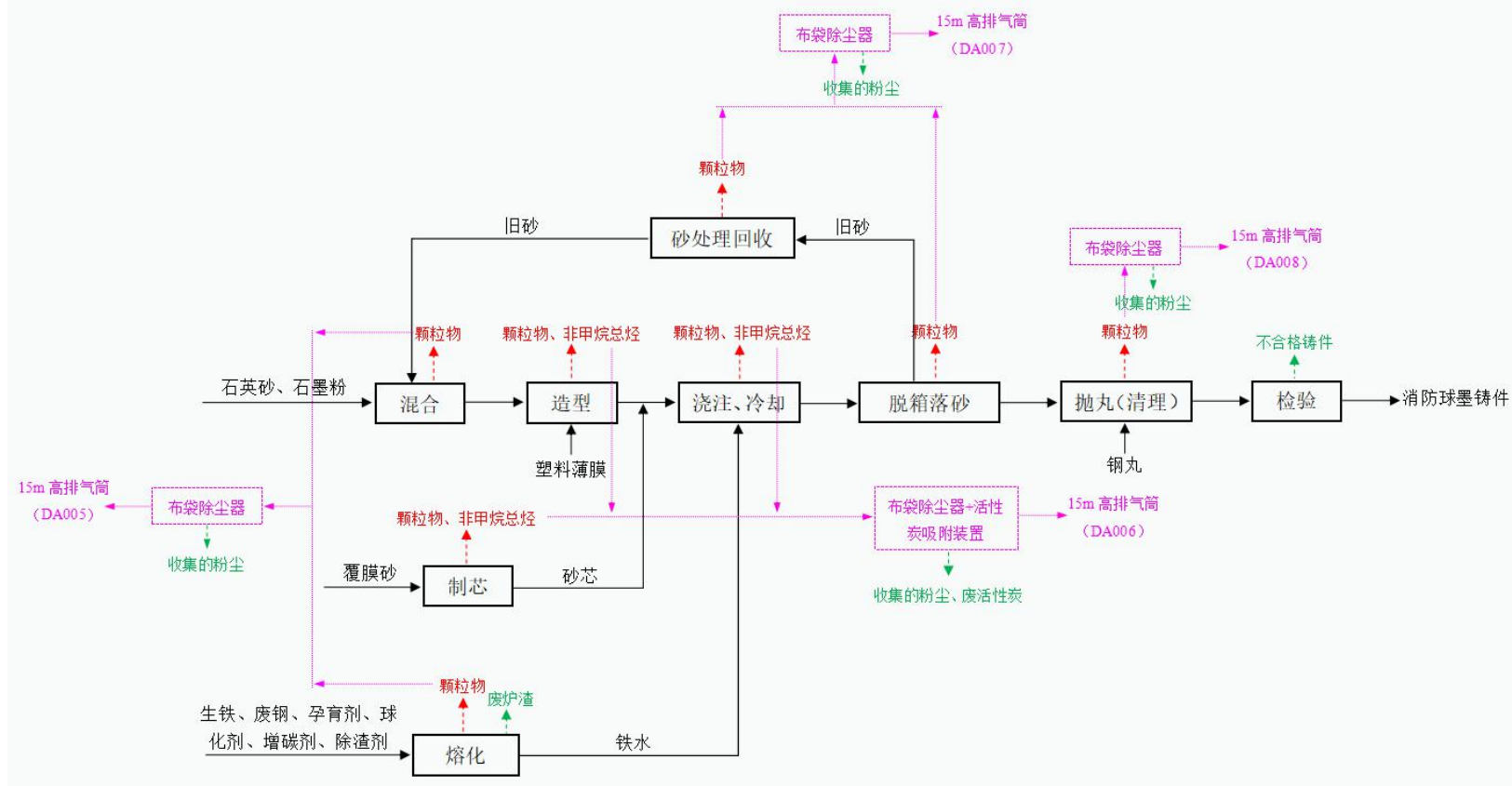
图 2-5 V 法铸造工艺及产污环节
