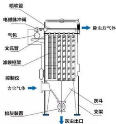
图 4-1 布袋除尘器示意图
